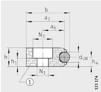
LFS...-FH
